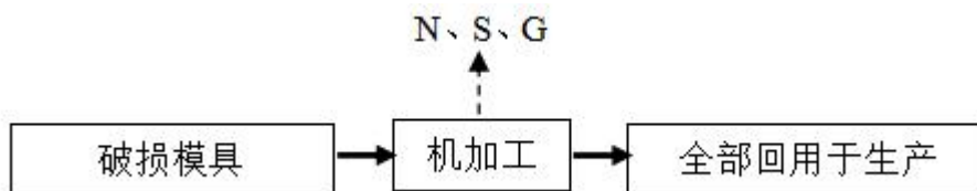
图 3-3 破损模具维修生产工艺及产污环节图
