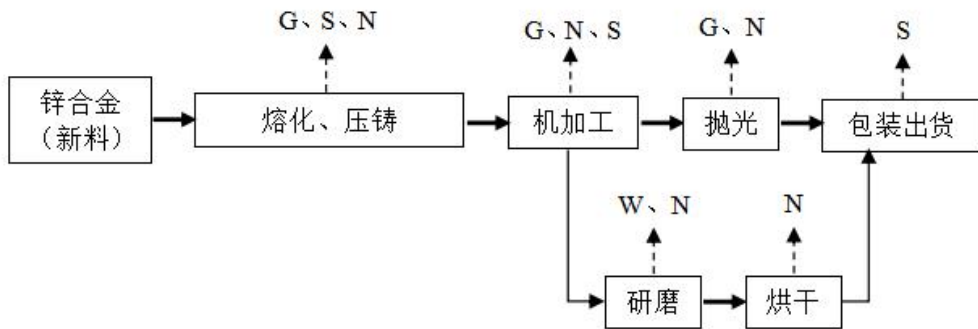
图 3-2 五金配件生产工艺及产污环节图
