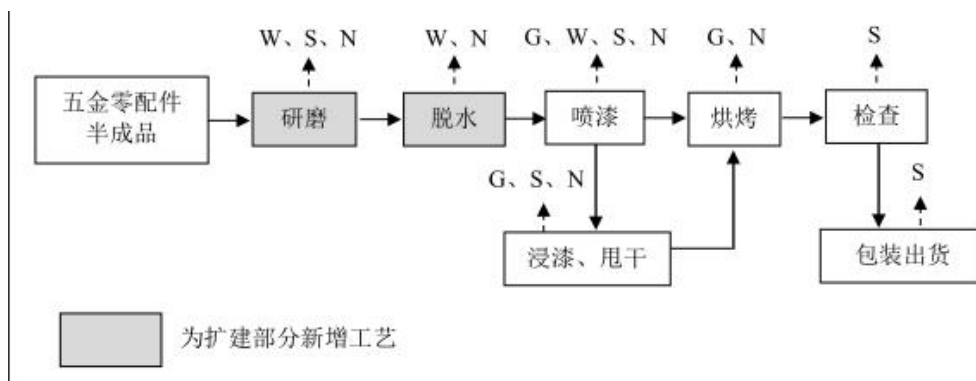
图 3-2 扩建项目五金零配件生产工艺及产污环节图
