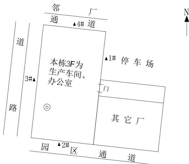
图 3-1 厂区平面布置及监测点位
