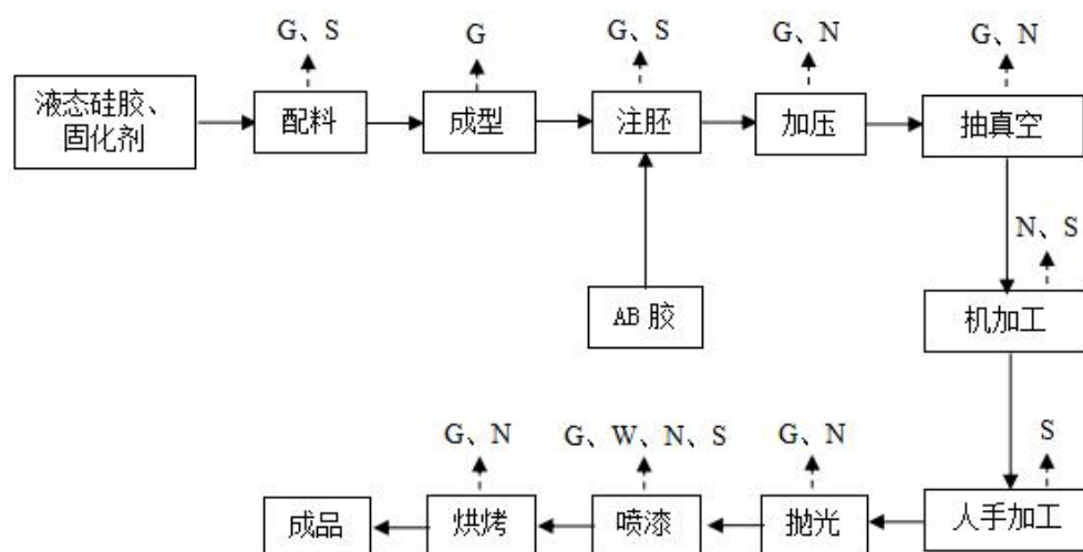
图 3-3 项目生产工艺及产污环节流程图
