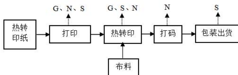
图 3-3 项目生产工艺及产污环节流程图
